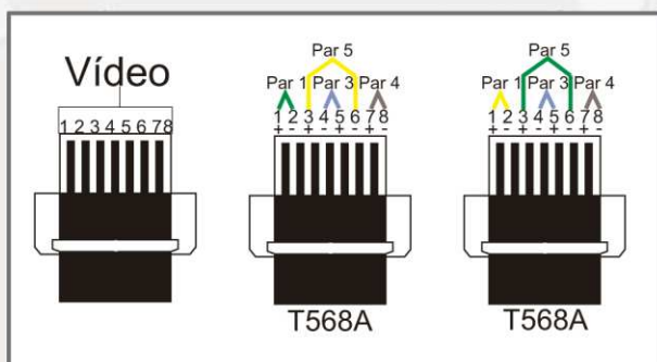
RJ-45 Fêmea (entrada do balun)
